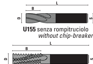
U156 con romptruciolo with chip-breaker
